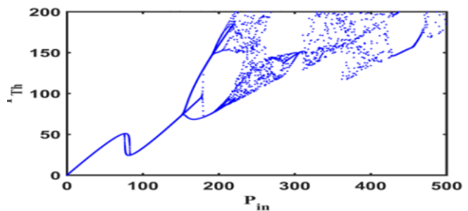
شکل ۳) نمودار شدت خروجی بر حسب شدت میدان از مشدد حلقوی دارای جفتگر الف) همسان \beta_1 = \beta_2 ب)
