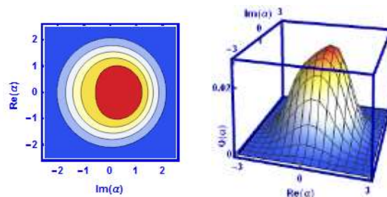
شکل ۲: تابع توزیع هوسیمی و نمودار کنتور متناظر با آن به ازای \lambda=3 و \zeta=0.5 ، \bar{n}=10 ، \alpha=x+iy
