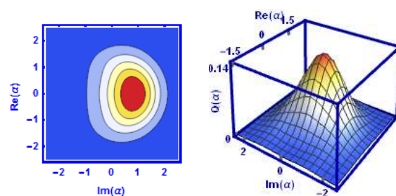
شکل ۱: تابع توزیع هوسیمی و نمودار کنتور متناظر با آن به ازای \lambda=3 و \zeta=0.5 ، \bar{n}=1 ، \alpha=x+iy
