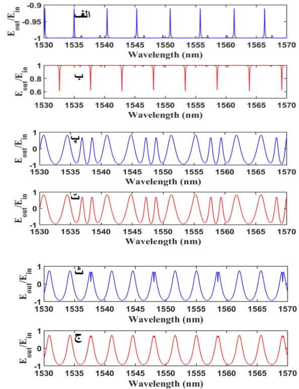
شکل ۳. نمودار نسبت میدانهای خروجی به ورودی در یک جفتگر 3 \times 3 خطی بر حسب طول موج با مقادیر جفتگری (الف) (K_{23}=0.59; K_{12}=0.2) (ب) (K_{23}=0.29; K_{12}=0.1) (K_{23}=0.615; K_{12}=0.885) (ت) (K_{23}=0.29; K_{12}=0.1) (K_{23}=0.25; K_{12}=0.82) (ج) (K_{23}=0.015; K_{12}=0.19) (ث)
