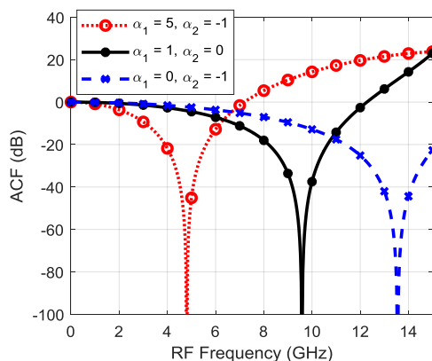
شکل ۲: تغییرات تابع ACF بر اساس تغییرات پارامتر chirp مدولاتورهای شدت نور
