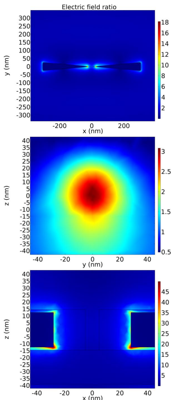
شکل ۲: توزیع دوبعدی میدان الکتریکی تقویت‌شده در اطراف نانو ساختاری از جنس طلا با روکش عایق و روی زیر لایه از جنس YAG در صفحه‌های xy و xz که از مرکز گاف نانو ساختار عبور می‌کنند.
