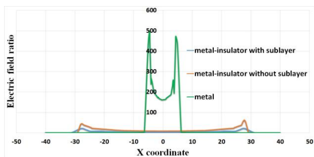
شکل ۳: توزیع یک‌بعدی میدان الکتریکی تقویت‌شده روی خط واصل بین دو رأس نانو ساختار ( z=0 ) برای حالت‌های نانو ساختار بدون روکش عایق، با روکش عایق و زیر لایه
