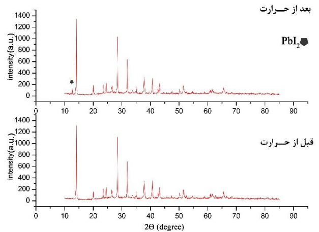
شکل ۴: نقش پراش XRD
