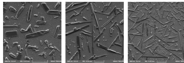
شکل ۴: تصویر SEM از لایه‌ی نازک اکسید مولیبدن رشد یافته با استفاده از روش الکتروشیمی. خط مقیاس به ترتیب از سمت چپ، ۱۰، ۱ و ۲۰ میکرون است.
