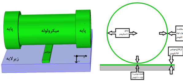
شکل ۱: شکل سمت راست: نمای سه بعدی طرحواره حسگر زیستی بر پایه تشدیدگر میکرولوله پیشنهادی و شکل سمت راست: برش عرضی در راستای X-Y در ناحیه ای از لوله که به موجبر تزویج شده است.
