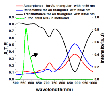
شکل ۶: منحنی طیف جذب (قرمز) و تراگیسل (سیاه) و بازتاب (آبی) برای بلور فوتونی و طیف فلورسانس رودامین- 6G (سبز).
