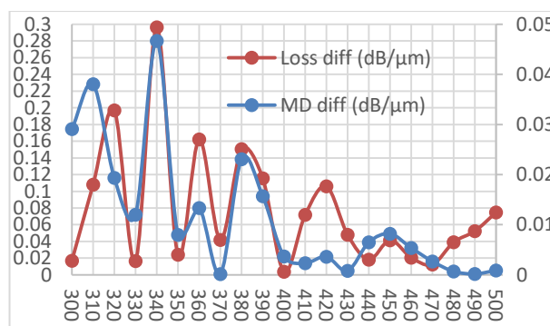
شکل ۵- اختلاف عمق مدولاسیون و اختلاف اتلاف بر حسب طول ضلع موجبر مربعی، محور سمت راست مربوط به اختلاف اتلاف و محور سمت راست مربوط به اختلاف عمق مدولاسیون می باشد.
