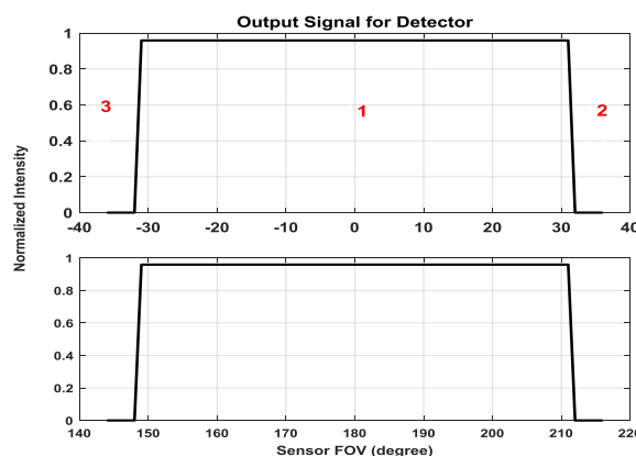
شکل ۶: پالس دریافتی از آشکارساز حسگر افق زمین.
