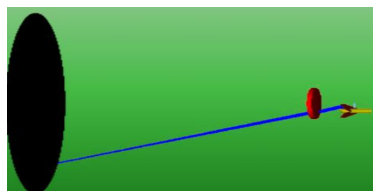
شکل ۵: نمای کلی شبیه سازی جهت تایید عدسی طراحی شده.
