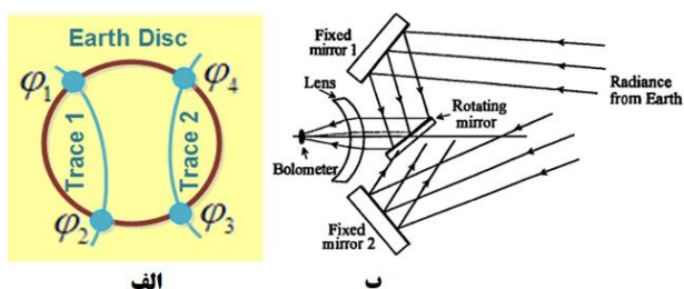
شکل ۱: الف: شمای کلی حسگر افق زمین اسکنینگ دوتایی [۵].
