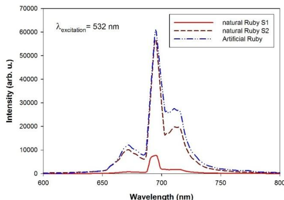
شکل ۷: طیف فلورسانس یاقوت (نمونه های طبیعی و مصنوعی) که با طول موج ۵۳۲ نانومتر تابش دهی شدند
