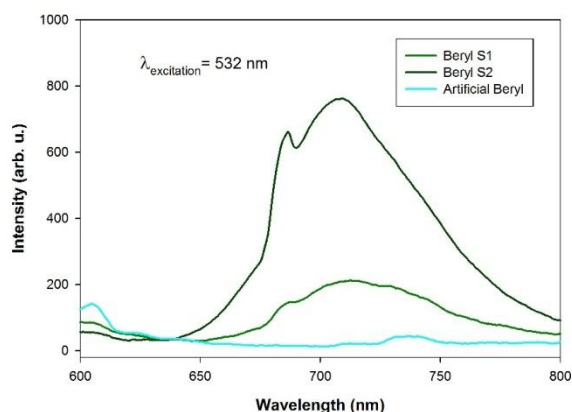
شکل ۶: طیف فلئورسانس زمرد (نمونه های طبیعی و مصنوعی) که با طول موج ۵۳۲ نانومتر تابش دهی شدند
