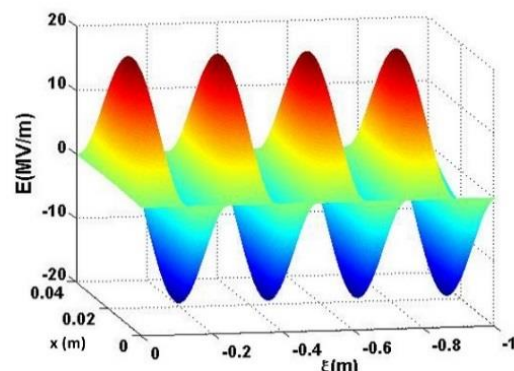
شکل ۲. توزیع میدان دنباله پالس در موجبر به عرض a = 4 \text{ cm} برای f = 5 \text{ GHz} , B = 1 \text{ mT} , I = 10^{10} \frac{\text{W}}{\text{m}^2}
