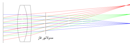
شکل ۱: نقشه‌ی لنز آکرومات با مدولاتور فاز
