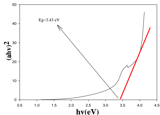
شکل ۴: نمودار تغییرات (\alpha h\nu)^2 بر حسب انرژی فوتون
