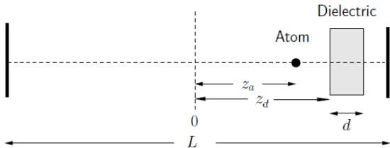
شکل ۱: شمایی از کاواک مورد بررسی. طول های مورد استفاده عبارتند از: z_d = 0.4L , z_a = 0.3L , d = 0.016L .
