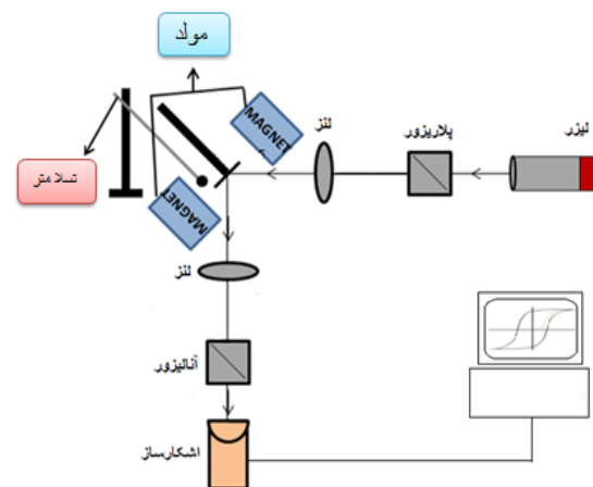
شکل ۶: چیدمان اثر مگنتو اپتیکی کر.
