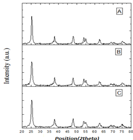
شکل ۱: الگوی XRD برای نانوذرات TiO 2 سنتز شده در pH مختلف: (A) pH=۱، (B) pH=۲ و (C) pH=۳.
