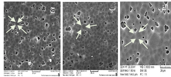
شکل ۲: تصاویر SEM میکروتخلخل‌های ایجاد شده روی سطح PMMA پس از تابش تک پالس با طول موج ۹۵۵۰ نانومتر با نرخ تکرار ۲ هرتز و در شاریدگی: الف) ۴۰۰۰، ب) ۸۰۰۰ و ج) ۱۲۰۰۰ میلی‌ژول بر سانتی‌متر مربع
