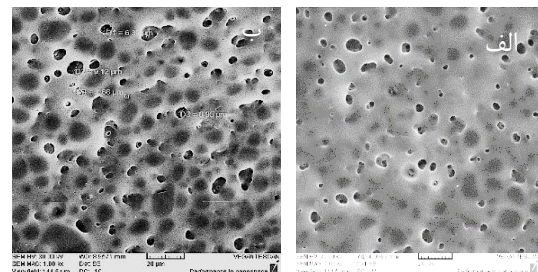
شکل ۳: تصاویر SEM میکروتخلخل‌های ایجاد شده روی سطح PMMA پس از تابش با طول موج ۹۵۵۰ نانومتر در شاریدگی ۲۰۰۰ میلی‌ژول بر سانتی‌متر مربع با نرخ تکرار ۱ هرتز و با تعداد پالس: الف) ۵۰ و ب) ۱۰۰
