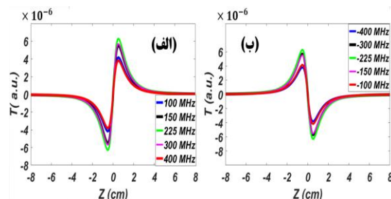
شکل ۲: تغییرات شدت عبوری بر حسب موقعیت بخار روبیدیوم نسبت به کانون.
