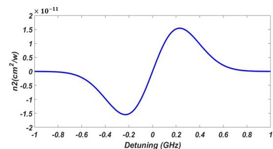
شکل ۱: تغییرات ضریب کر بر حسب واوکوی‌های مختلف نسبت به فرکانس تشدید.
