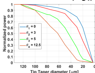
شکل ۵: توان منتشر شده در طول TTF بر اساس چهار زاویه ی مختلف تزویج نور به درون فیبرنوری
