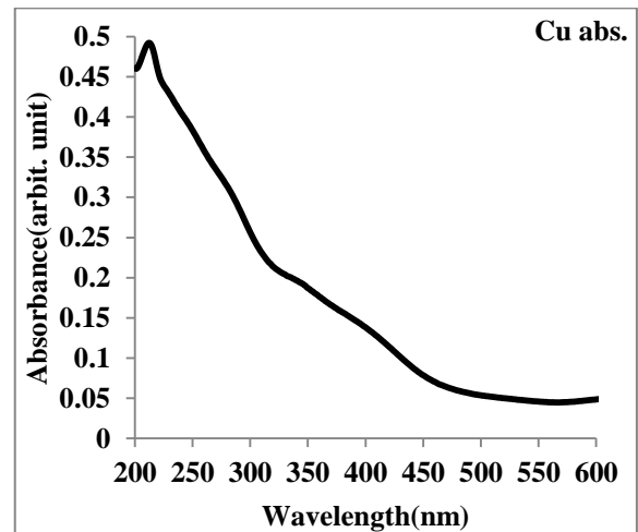
شکل ۵: بیناب جذب نوری محلول نانوذرات مس.
