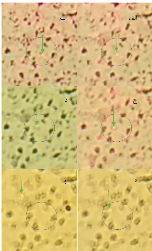
شکل ۶: الف، ب، ج مکان ذره به ترتیب ۲:۰۰، ۲:۰۱، ۲:۰۲ و ۲:۰۳ دقیقه بعد از روشن شدن لیزر. د، ه، و مکان ذره هنگام آزاد شدن از تله به ترتیب در لحظه خاموشی لیزر، ۱۷، ۳۴، ۳۵ ثانیه بعد از خاموشی لیزر، مدت زمان ماندن در تله ۲:۰۲ ثانیه
