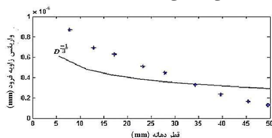
شکل ۳: تغییرات واریانس زاویه فرود بر حسب قطر دهانه‌ی پرتو
