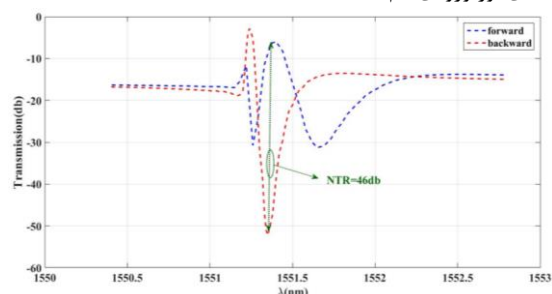
شکل ۴. طیف عبور رفت و برگشت برای ساختار شکل ۱(ب) هنگامی که دامنه ی میدان الکتریکی ورودی 1.1 \times 10^8 V·m -1 است.
