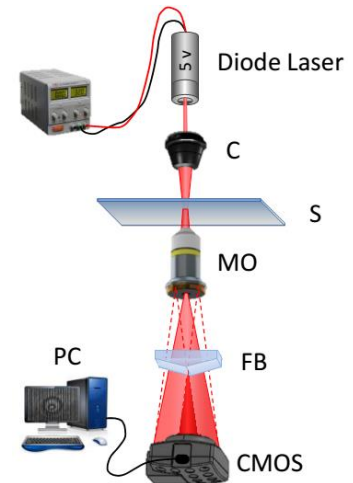
شکل ۲: چیدمان آزمایش. C چگالنده، MO عدسی شیئی میکروسکوپ، S نمونه، و FB دومنشور فرنل هستند.
