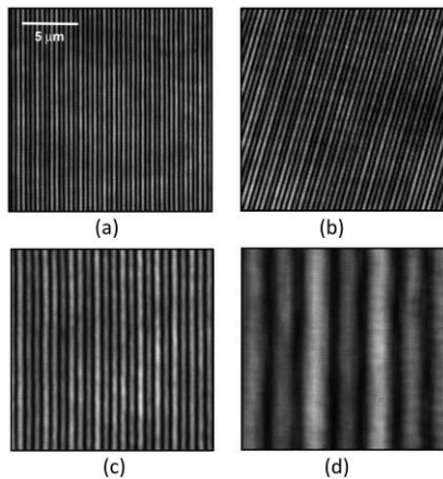
شکل ۳: تمام‌نگاشت‌های ثبت شده در فواصل متفاوت دومنشور نسبت به دوربین، (a) a=8 cm، (b) به ازای چرخش 25 درجه دومنشور حول محور z ، (c) a=12 cm، (d) a=16 cm.
