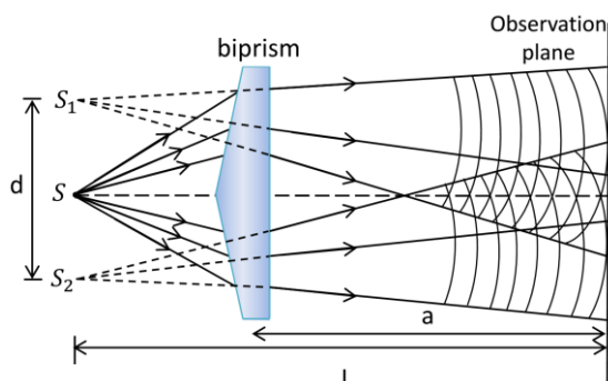
شکل ۱: هندسه‌ی تشکیل فریزهای تداخلی در دو منشور فرنل.
