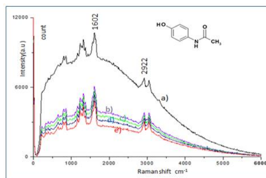
شکل ۲- طیف رامان قرص استامینوفن پس از (a) t=0 و (b) t=20 ، (c) t=30 ، (d) t=40 و (e) t=60 دقیقه تاباندن نور لیزر به نمونه
