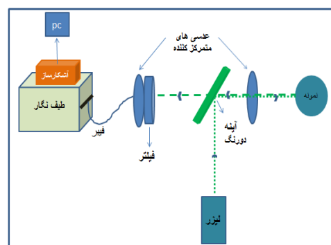
شکل ۱- چیدمان آزمایشگاهی برای طیف سنجی رامان
