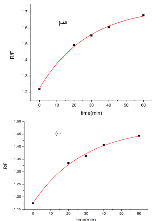
شکل ۳: نمودار نسبت سیگنال رامان به زمینه‌ی فلورسنس برای (الف) پیک 1602\text{ cm}^{-1} و (ب) پیک 2922\text{ cm}^{-1} برای نمونه‌ی قرص استامینوفن
