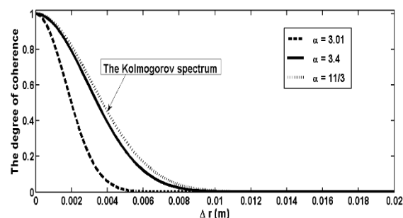
شکل ۱: تغییرات درجه طیفی همدوسی باریکه PCFT در حال انتشار در اتمسفر متلاطم غیر کولموگروف برای مقادیر مختلف \alpha
