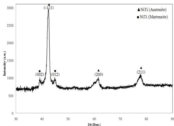
شکل ۲. الگوی پراش اشعه ایکس از آلیاژ پایه نایتینول که در آن ▲ نشان دهنده‌ی فاز آستنیت آلیاژ نایتینول و ■ بیانگر فاز مارتنزیت آلیاژ نایتینول می‌باشد.
