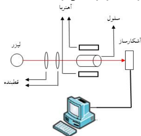
شکل ۴: چیدمان اندازه‌گیری ترازیهای زیمن با استفاده از نور قطبیده خطی
