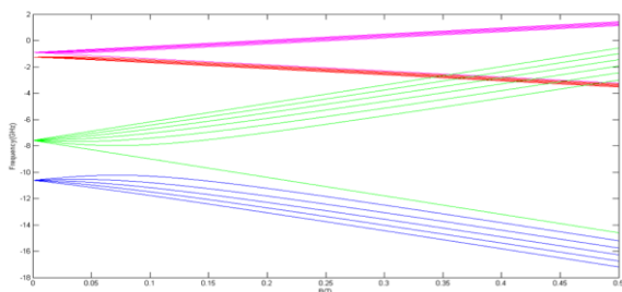
شکل ۲: ساختار فوق‌ریز ترازیهای مربوط به گذار D_1 روبیدیوم ۸۵ در حضور میدان مغناطیسی خارجی
