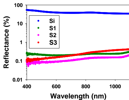
شکل ۵: طیف بازتاب سیلیسیم کپه ای و نانو سیم‌های سیلیسیم تهیه شده در زمان‌های مختلف.
