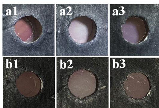
شکل ۶- لایه‌ی Ag-AgCl (a) قبل از تابش نور سفید و (b) بعد از تابش نور سفید. نقاط a1 و b1 با پرتوهای لیزر هلیوم-نئون، a2 و b2 با لیزر Nd:YAG و a3 و b3 با لیزر دیودی بنفش نوردی شده است.
