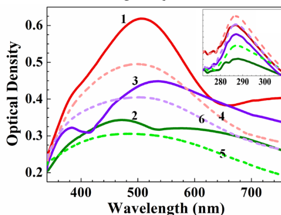
شکل ۷- بیناب جذب لایه‌ی نازک Ag-AgCl قبل از اینکه تحت تابش نور سفید قرار گیرد که به ترتیب 1، 2 و 3 با لیزرهای هلیوم-نئون، Nd:YAG و دیودی بنفش نوردی شده است. با همین ترتیب 4، 5 و 6 بیناب جذب نمونه‌ها بعد از تابش نور سفید است.
