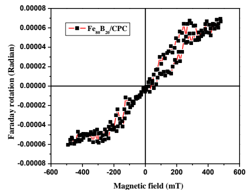
شکل ۵ - نمودار تغییرات شدت FR در دمای اتاق از نمونه Fe_8B_2/CPC
