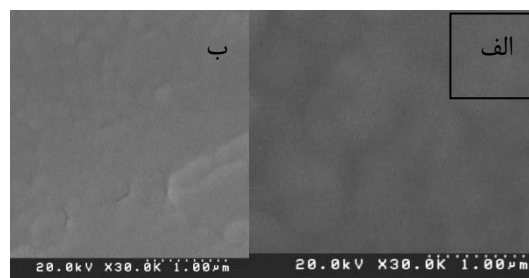
شکل ۳. تصویر FE-SEM از نمای بالای لایه الف) Fe_8B_2 ب) BFO روی CPC.
