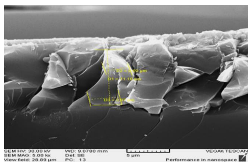
شکل ۵- مقطع عرضی از سطح نانوتیوب های سوزنی شکل
