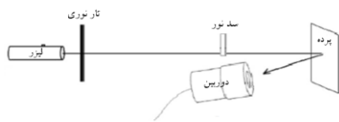
شکل ۴: نحوه‌ی قرارگیری سد نور در سر راه نور پراشیده شده از تار نوری.
